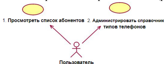
Рисунок 1 – Варианты использования телефонной книги
